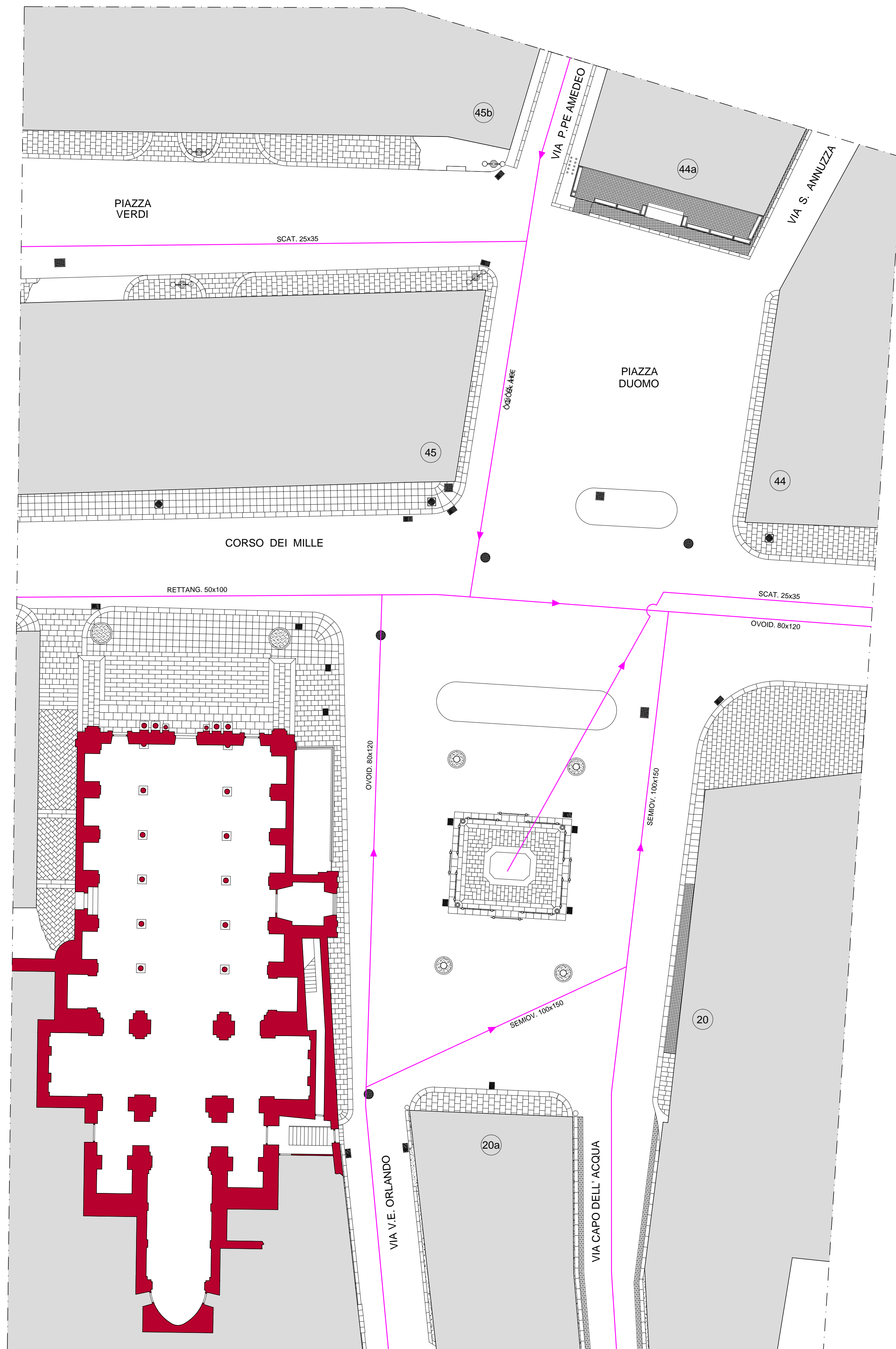
PLANIMETRIA GENERALE DELLA RETE FOGNANTE STATO ATTUALE
